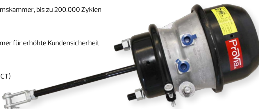
Doppelmembranbremszylinder Nocken
