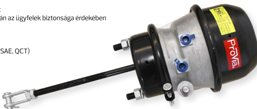
Dupla membrános rugóerő-tárolós fékmunkahenger cam
