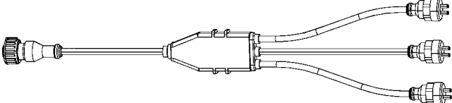
472 880 928 2 Adapterkábel (háromutas)
